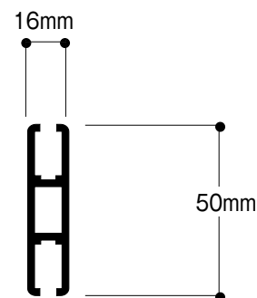
ビーム断面図
