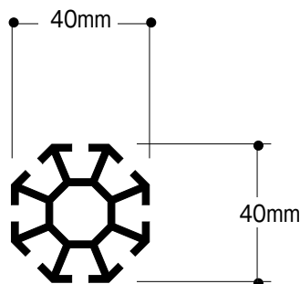
ポール断面図
